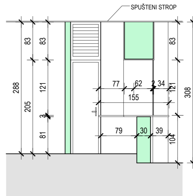
PRESJEK - NOVO STANJE
