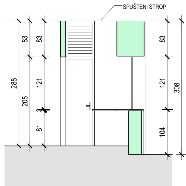
PRESJEK - POSTOJEĆE STANJE
