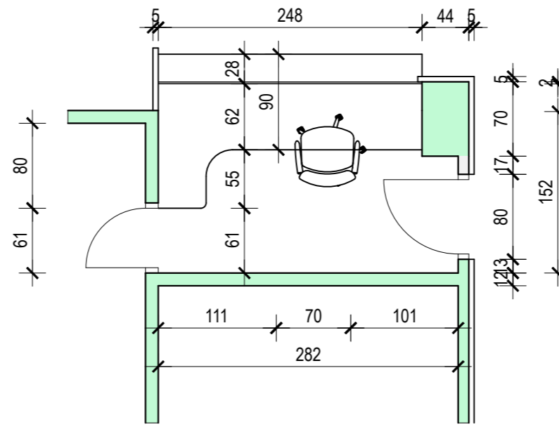
TLOCRT - NOVO STANJE
