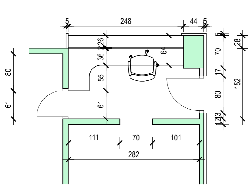
TLOCRT - POSTOJEĆE STANJE
