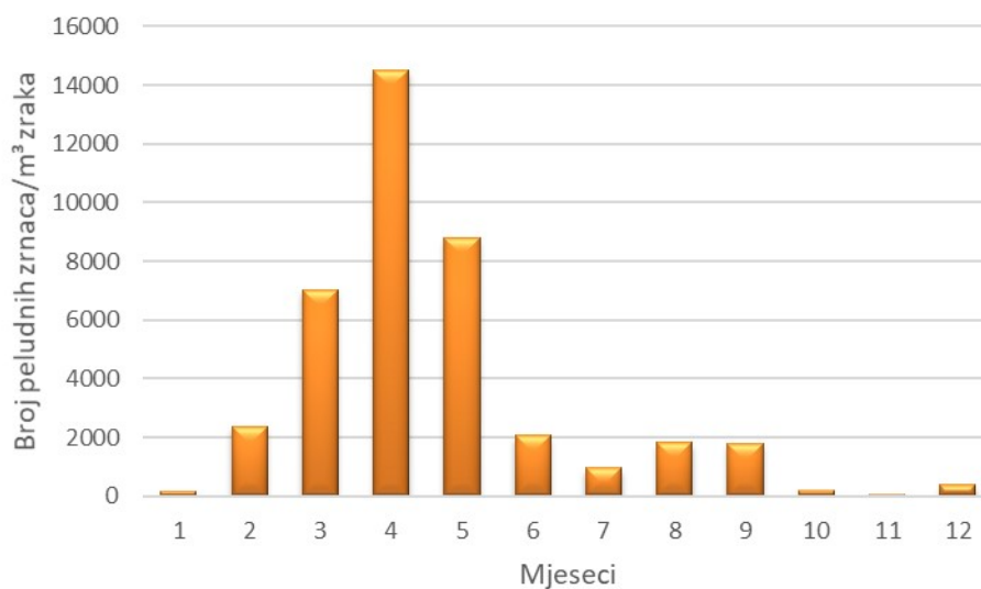
Slika 4. Mjesečne varijacije koncentracija peludi u zraku grada Rijeke u 2023. godini.
