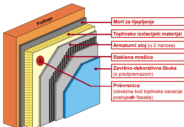
Struktura povezanog sustava za vanjsku toplinsku izolaciju (ETICS)
